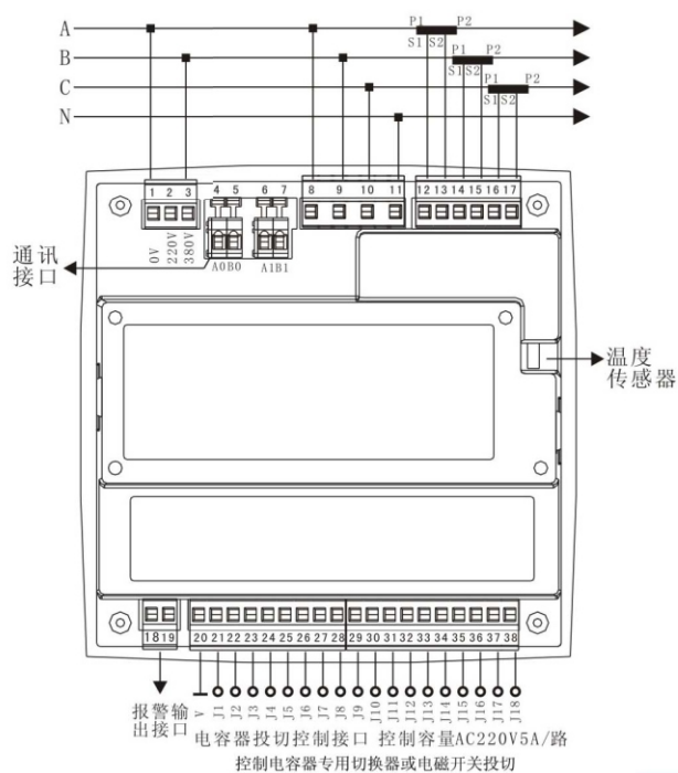
VPFC5-18C型控制器接线图(静态输出)电源取380V
