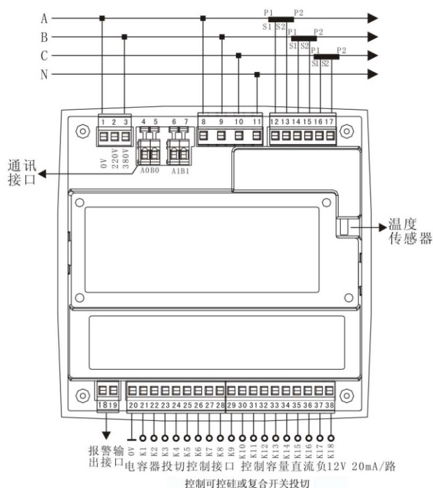
VPFC5-18D型控制器接线图(动态输出)电源取380V
