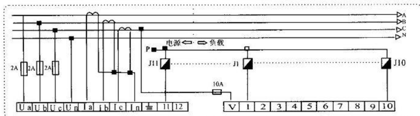
VPFC3-12型开孔尺寸为113mm×113mm接线图 静态输出（建议匹配VCJR型电容专用切换接触器） 当接触器额定工作电压为220V时P点接N，380V时P点接B；
