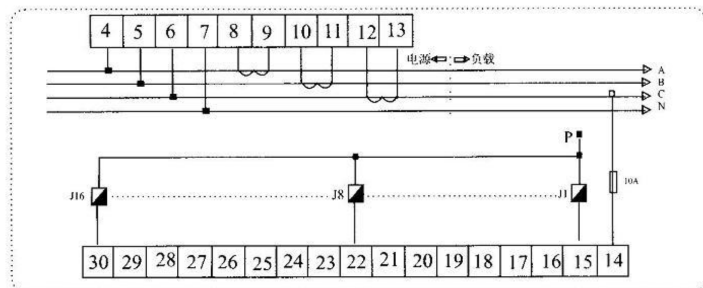
VPFC3-16F型开孔尺寸为138mm×138mm接线图 静态输出（建议匹配VCJR型电容专用切换接触器） 当接触器额定工作电压为220V时P点接N，380V时P点接B；
