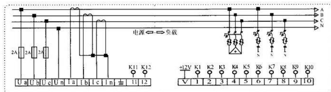
VPFC3-12-D型开孔尺寸为113mm×113mm接线图 动态输出 (建议匹配VKCS型无触点调节器或VEK型复合投切装置)
