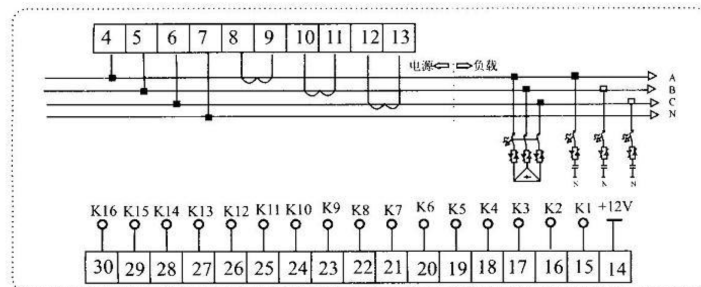
VPFC3-16F-D型开孔尺寸为138mm×138mm接线图 动态输出 (建议匹配VKCS型无触点调节器或VFK型复合投切装置)
