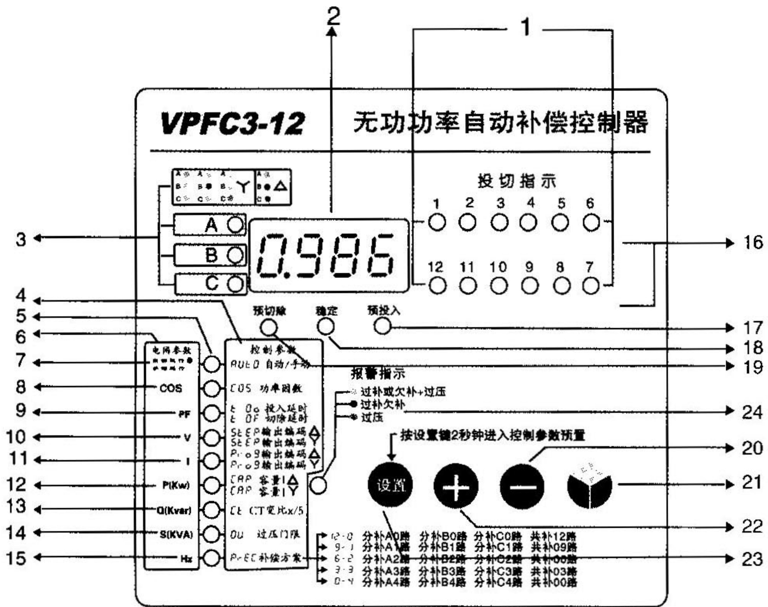
VPFC3-12型（开孔尺寸113mm×113mm）控制面板功能图
